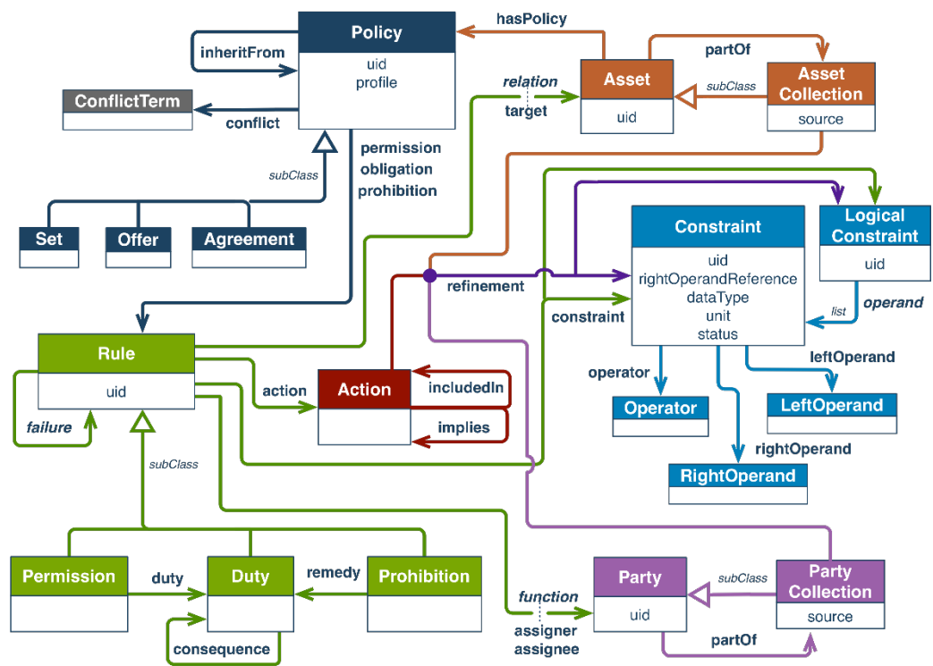
Afbeelding van een deel van het ODRL model. Bron: https://www.w3.org/TR/odrl-model/
